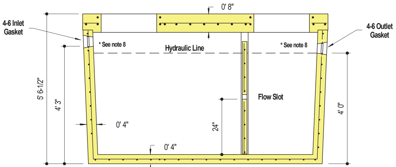
SECTION A-A
