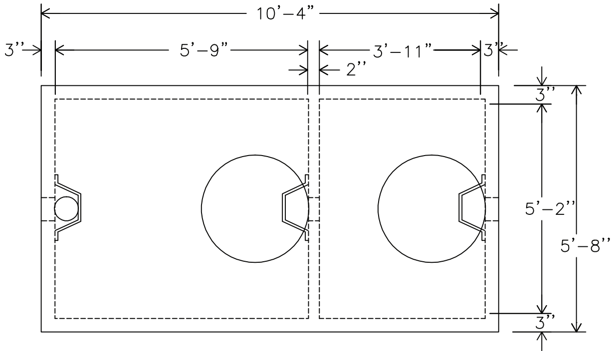
—PLAN—
