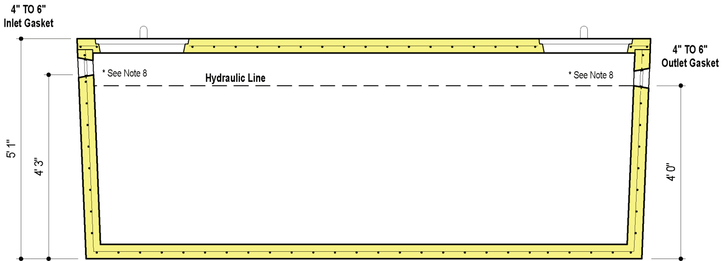
SECTION A-A
